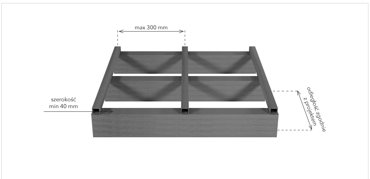
Rys 3. Legary na konstrukcji stalowej
