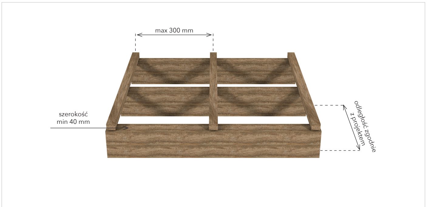
Rys 2. Legary na konstrukcji drewnianej
