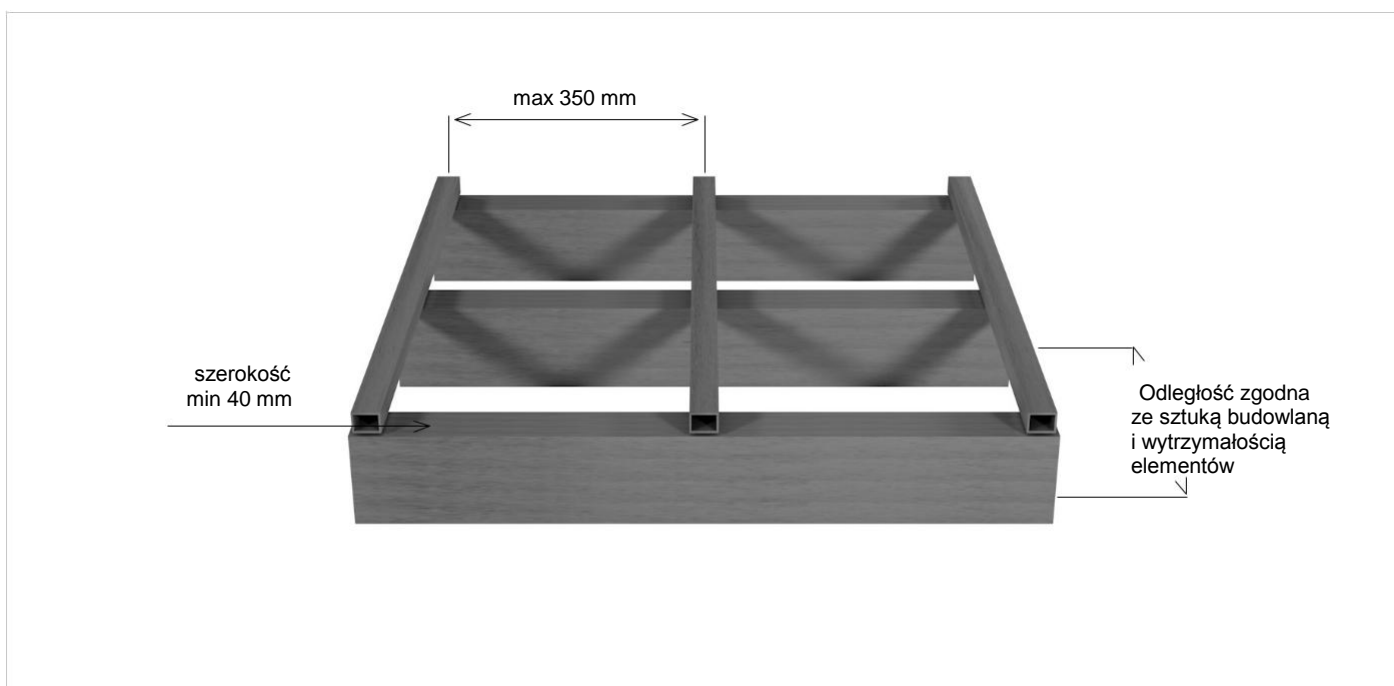
Rys 3. Legary na konstrukcji stalowej
