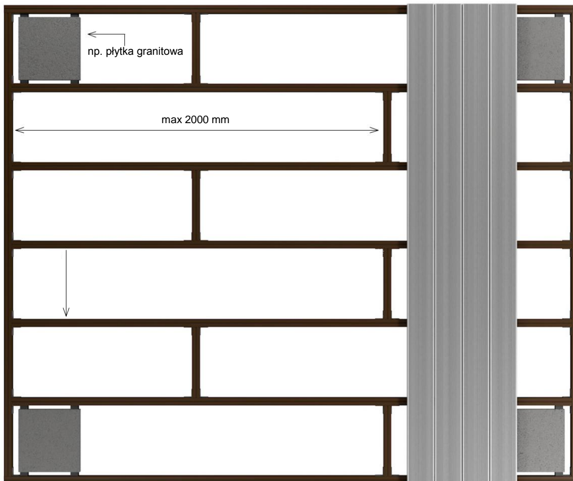
Rys 7. Taras pływający - rama z legarów połączona kątowymi łączami ciesielskimi, obciążona płytami betonowymi
